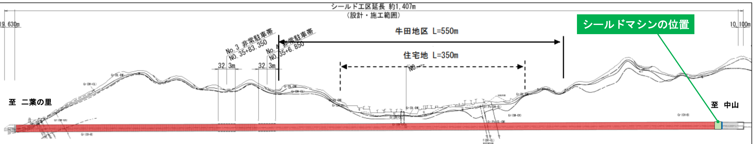
縦断図
