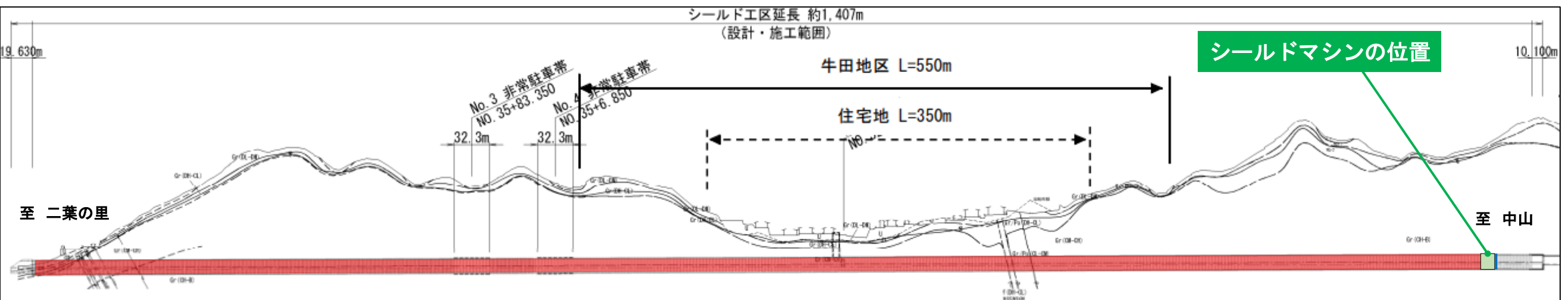
縦断図
